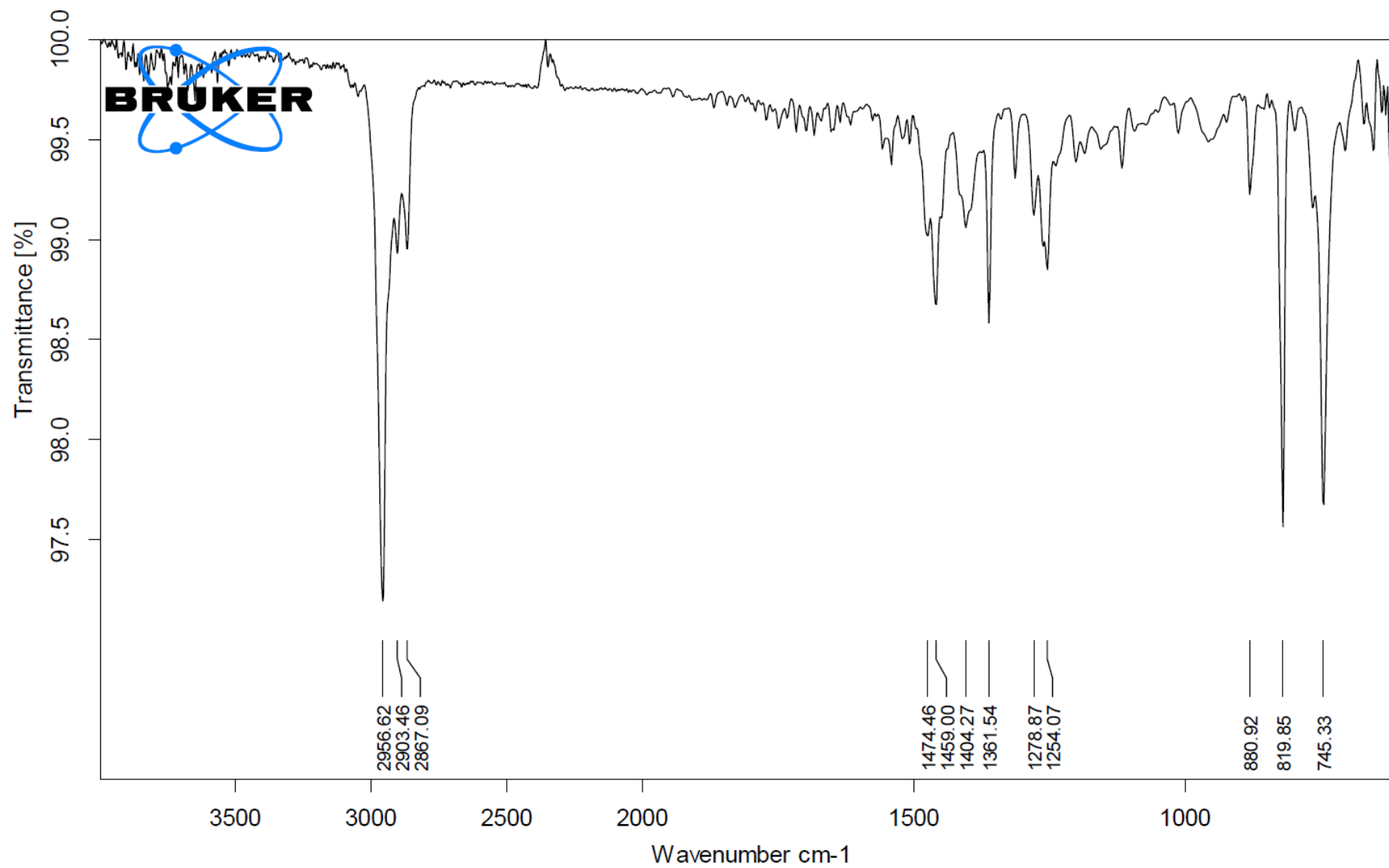
IR of t Bu-MsFluidBr (4)
